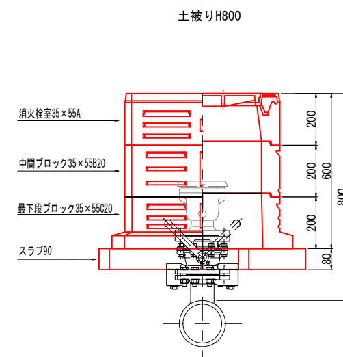
空気弁室設置標準図
