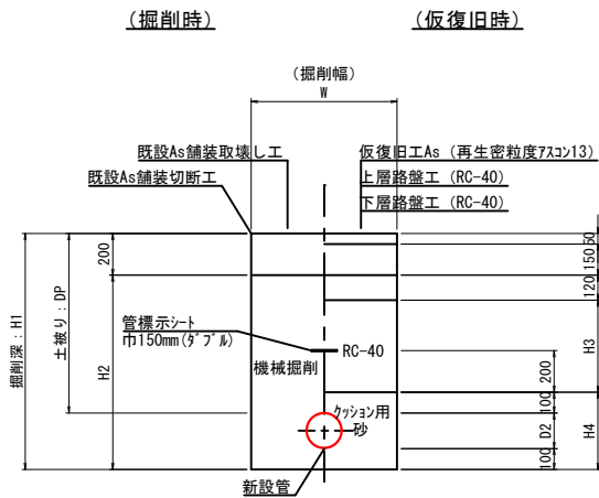
新設管布設土工 車道部(県道)
