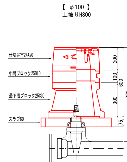
排泥弁室設置標準図
