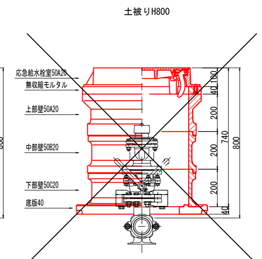
応急給水栓室設置標準図
