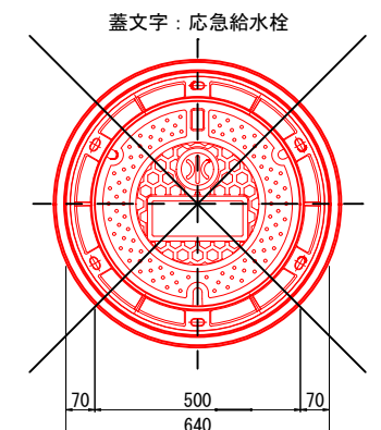
丸型50蓋付枠応急給水栓
