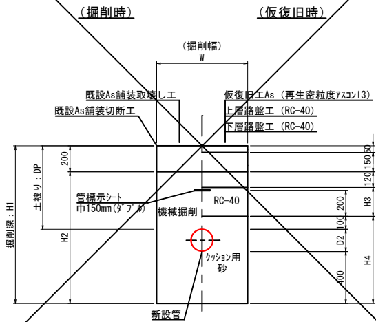
新設管布設土工 不断水分岐部(県道)
