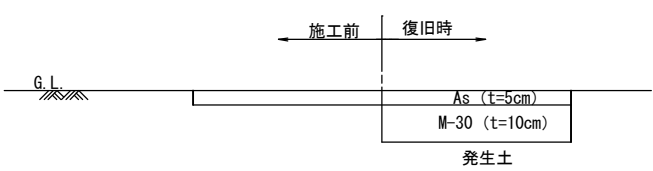
ハンドホール周辺断面図
