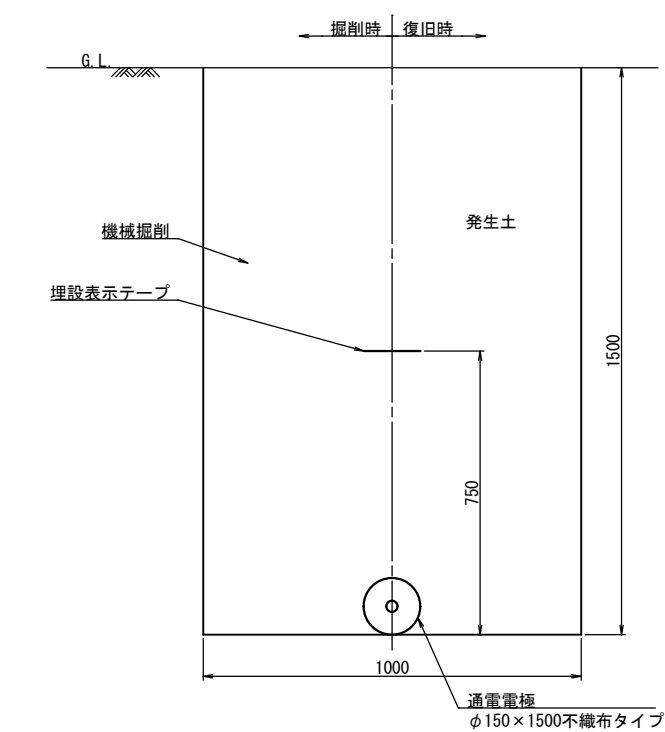
A-A' 通電電極設置部断面図
