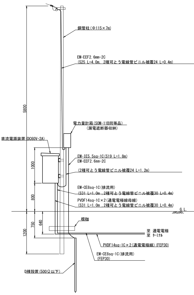
C-C' 直流電源装置断面図
