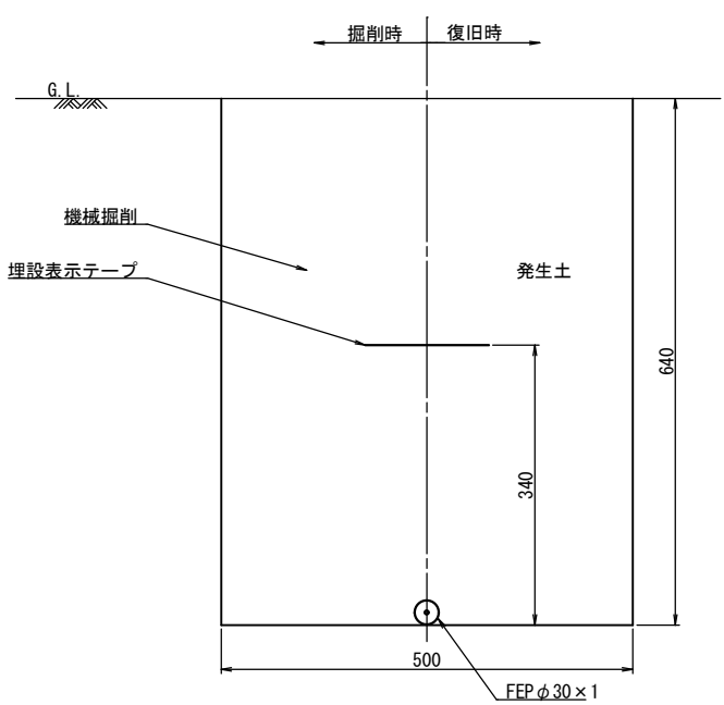
B-B' 電線管掘削部断面図
