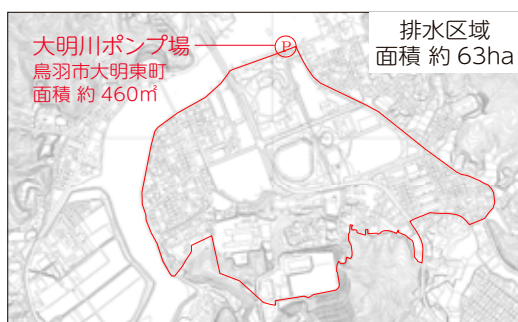
鳥羽公共下水道（雨水）計画図
