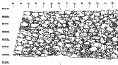
石垣立面図
