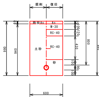
配水管(2号土工) HPE \phi 75
