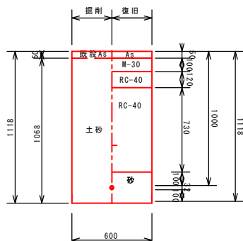
給水引込管(5号土工) HIVP \phi 25
