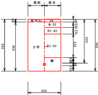
配水管 (9号土工 HIVP \phi 40 )
