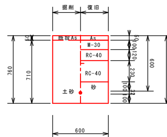
配水管(4号土工) HIVP \phi 25
