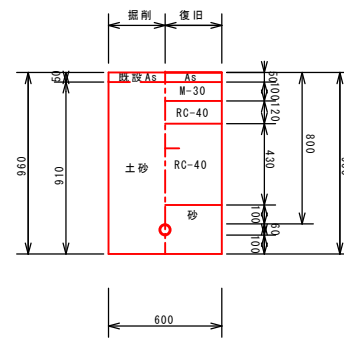
排泥管(7号土工) HIVP \phi 50
