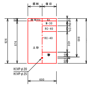
配水管 (3号土工) HIVP \phi 25 \cdot \phi 20
