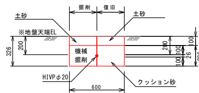
給水引込管(宅内) HIVPφ20 (8号土工)
