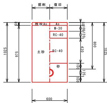
配水管(1号土工) HPE \phi 100
