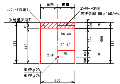
給水引込管(6号土工) HIVP \phi 25 \cdot \phi 20
