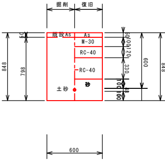
管(10号土工 HIVP \phi 40
