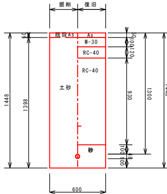
込管(11号土工 HIVP \phi 40
