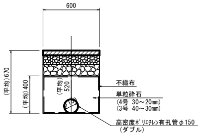
暗渠排水管 (B)
