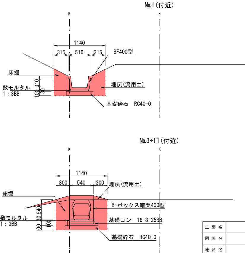
標準断面図
