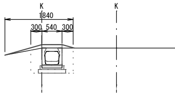
No.3+11.8(同所) FH=1.56 GH=1.47
